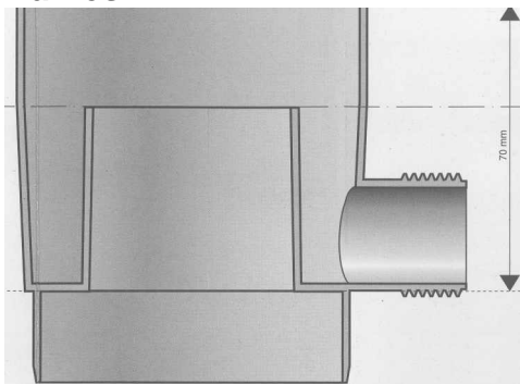
Ilustrační obrázek – sběrač dešťové vody DN75
